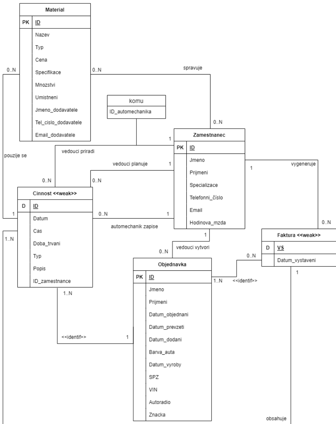
Obr. 2: ER Diagram
