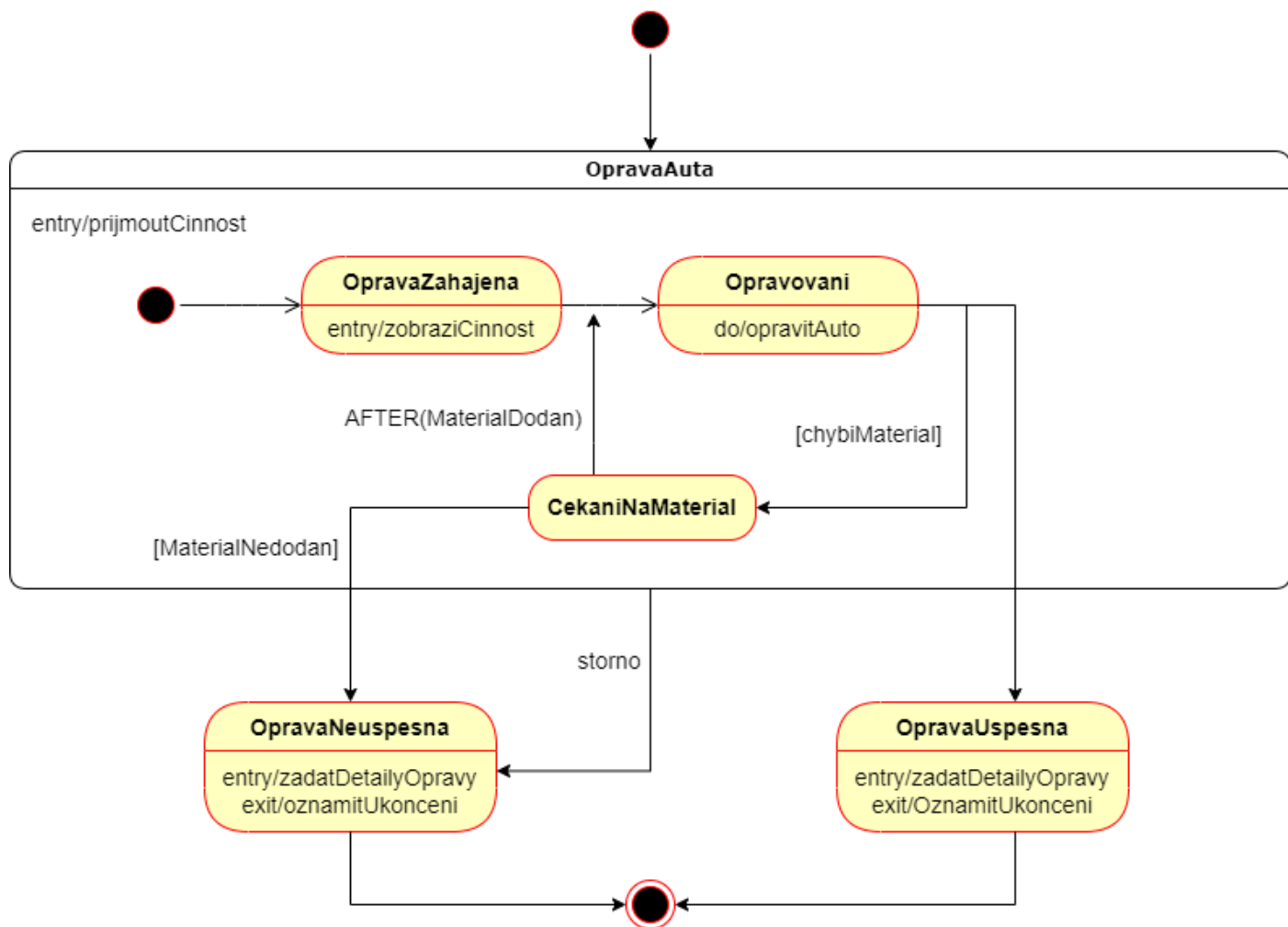
Obr. 6: Stavový diagram
