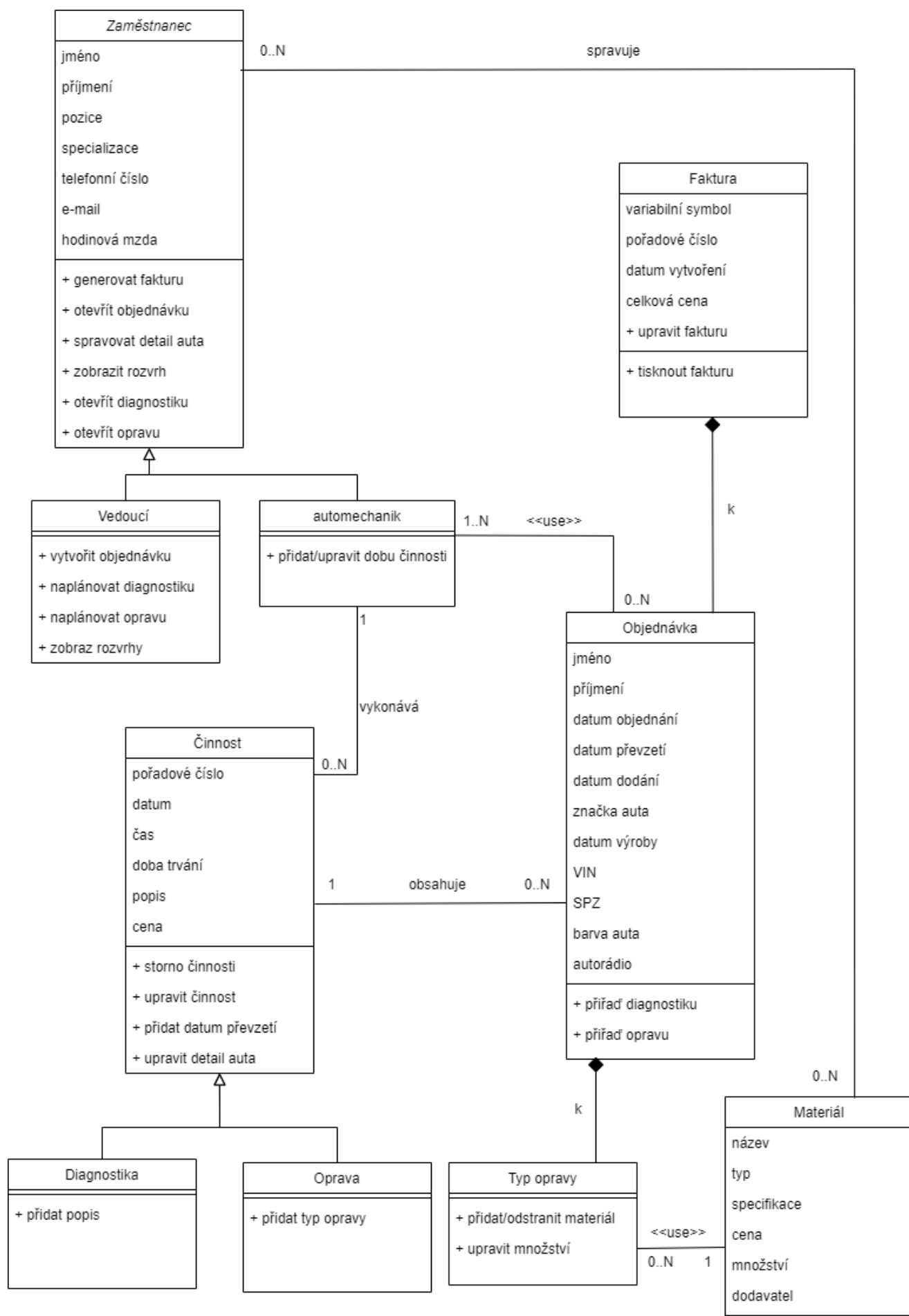
Obr. 3: Diagram tříd
